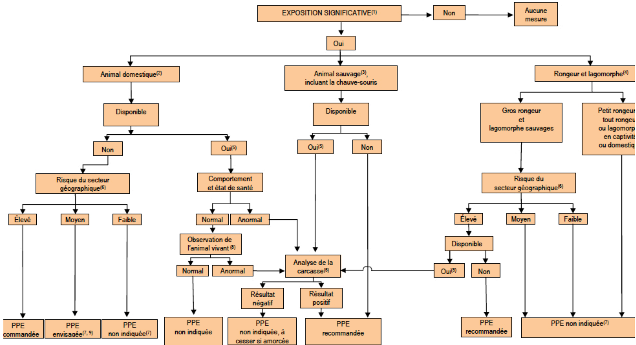
Figure 3 : Algorithme d'aide à la décision pour la PPE contre la rage
